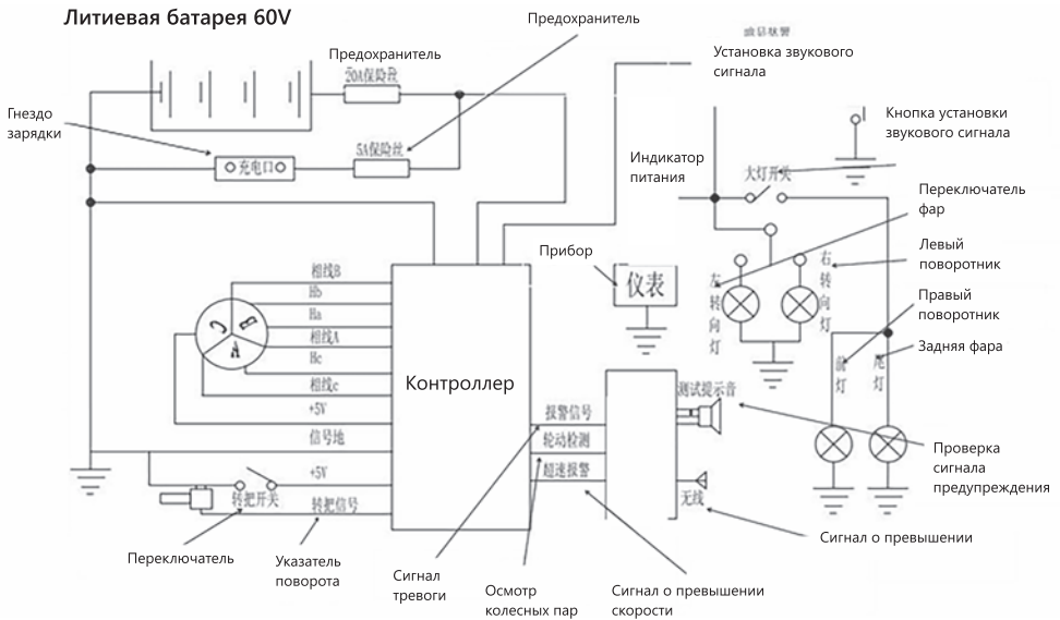
Схематический чертеж электроприбора
